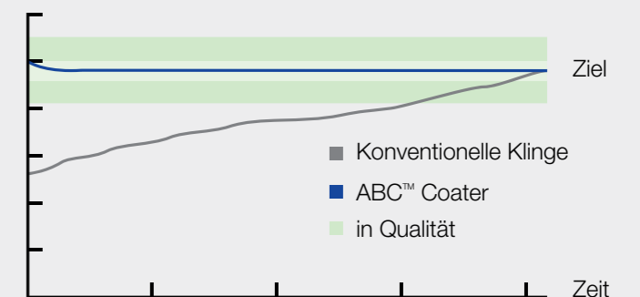
Diagramm zeigt die Reproduzierbarkeit des ABC™ Systems. Die Einstellungen der vorangegangenen Produktion sind nach wie vor gültig.
