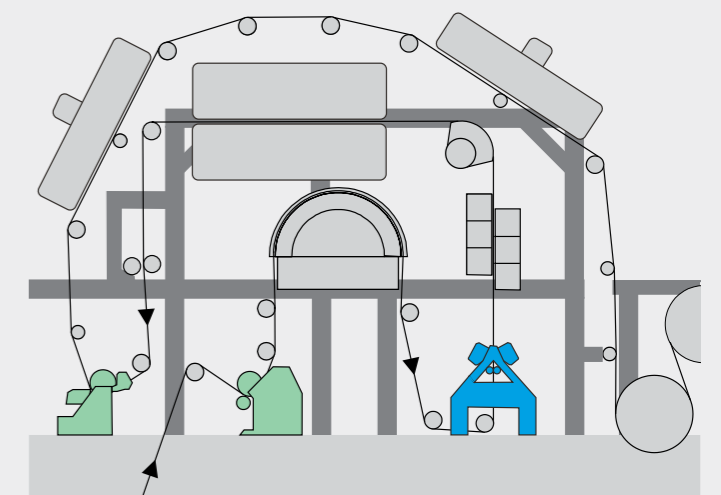
Künftig: 2+2 Strichlagen beim selben Platzbedarf in der Maschine
